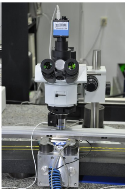
Fragment stanowiska pomiarowego do wzorcowania wzorców kreskowych
