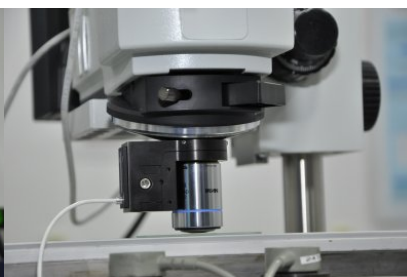
Fragment stanowiska pomiarowego do wzorcowania wzorców kreskowych
