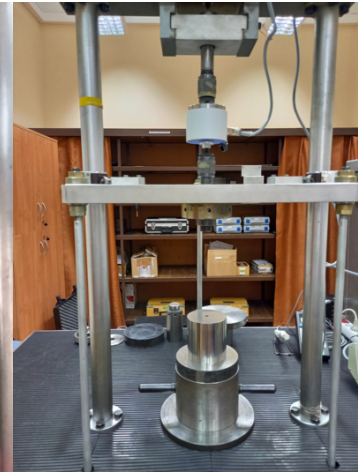
maszyna wzorcowa siły
